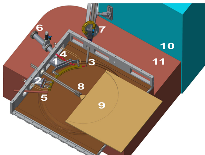
Model uspořádání shlukovacího systému v komoře cyklotronu U-120M. 1 – první deflektorová sekce, 2 – druhá deflektorová sekce, 3 – přebíjecí folie, 4 – trajektorie svazku po přebití, 5 – integrální sonda č. 3, 6 – pozice Be terče, 7 – integrální sonda č. 2, 8 – PIG iontový zdroj, 9 – duant, 10 – magnet cyklotronu, 11 – hlavní vlnutí cyklotronu.
