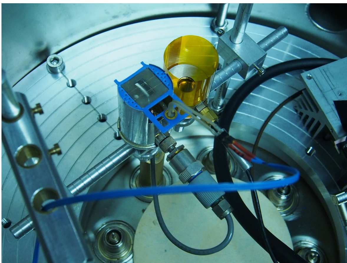
Pohled na experimentální uspořádání ve vakuové komoře metody neutronového hloubkového profilování NDP. Vzorek baterie (uchycený v modrém rámečku) je umístěn v držáku nad detektorem nabitých částic.
