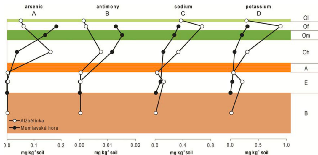
Hloubkové profily obsahu As, Sb, Na a K v půdních lipidech ze studovaných půdních horizontů.
